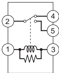
Fan control relay
