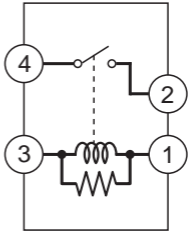
Condenser fan relay
