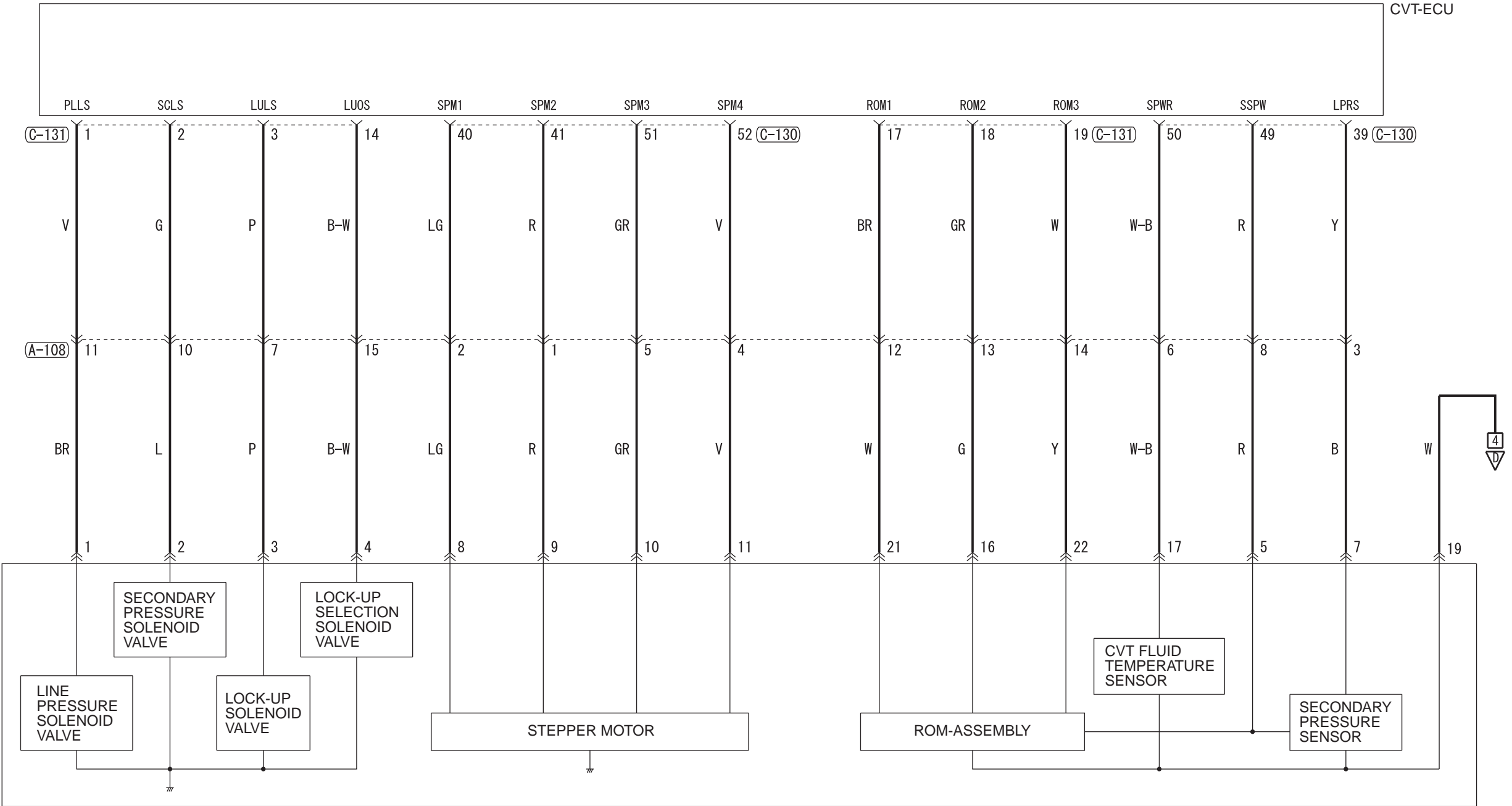
CVT ASSEMBLY (B-108)
