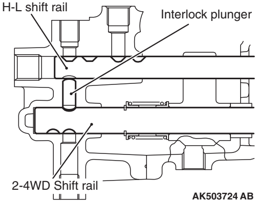
2-4WD Shift rail
