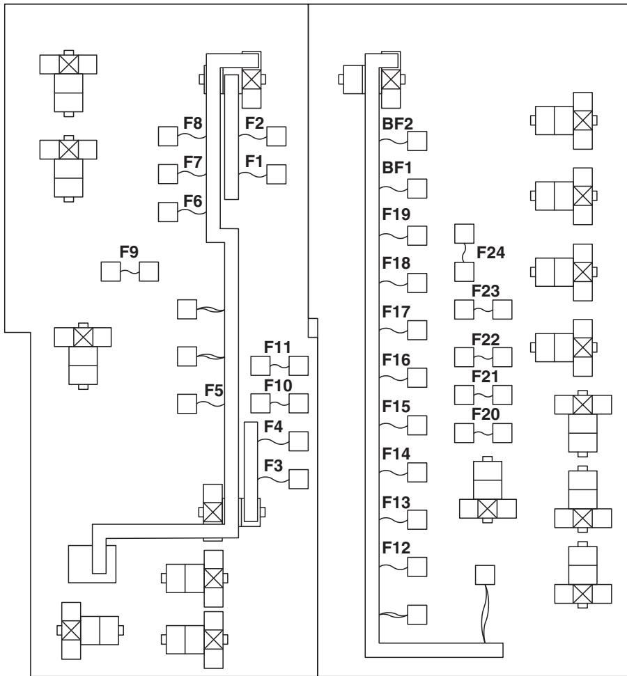
Relay box fuse No.BF1, BF2, F1 to F24
